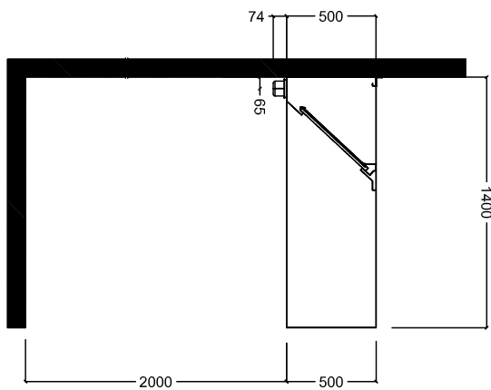
Zij aanzicht
